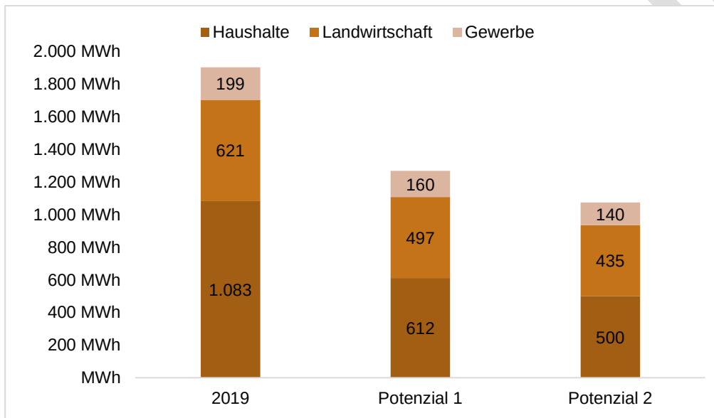
Abbildung: Stromeinsparpotenziale im Quartier (eigene Berechnungen)
