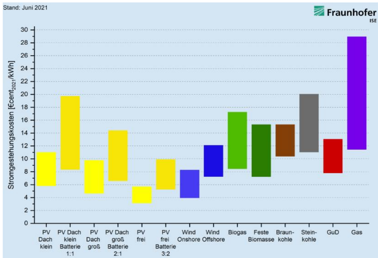
Abbildung: Stromgestehungskosten für erneuerbare Energien und konventionelle Kraftwerke an Standorten in Deutschland 18
