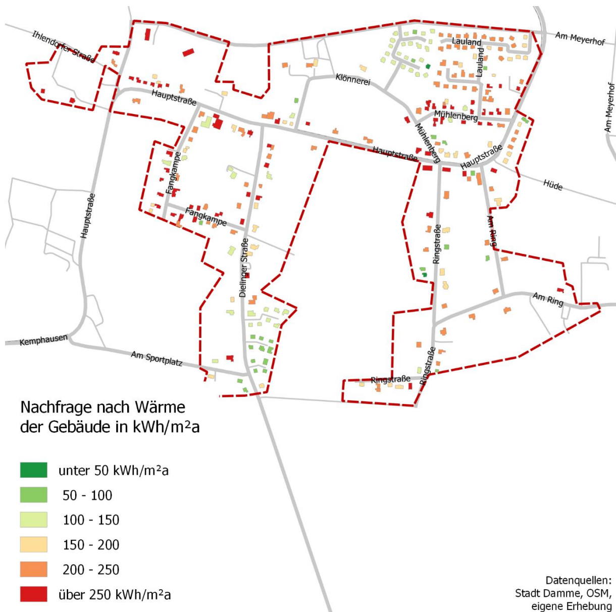
Abbildung 2: Nachfrage nach Wärme der Gebäude in kWh/m²a
