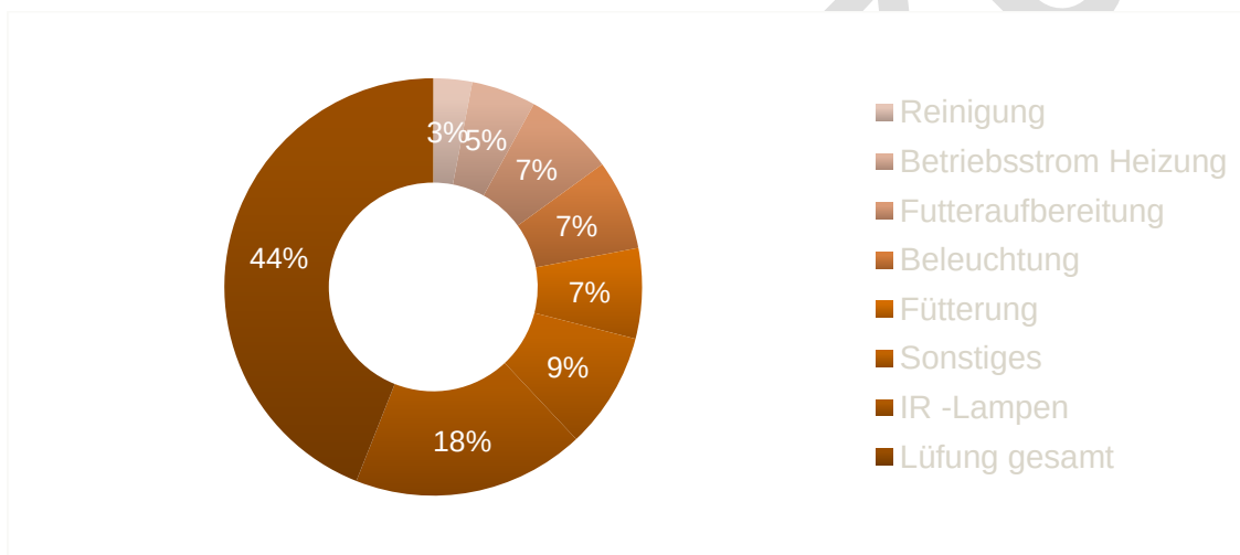
Abbildung: Verteilung des Stromverbrauchs am Beispiel von spezialisierten Ferkelerzeugerbetrieben 14
