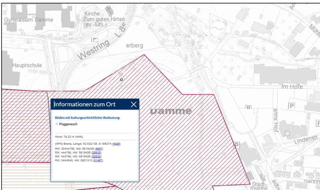
Abb. 7: Suchraum für schutzwürdige Böden (BK50 NIBIS Kartenserver)
